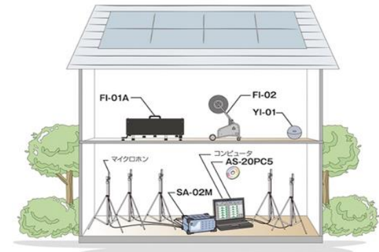
騒音・振動実験
