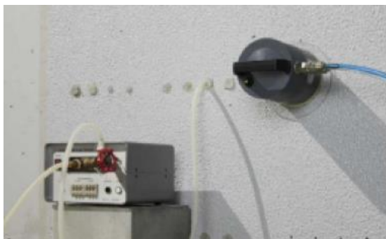
ダブルチャンバー法での測定状況
