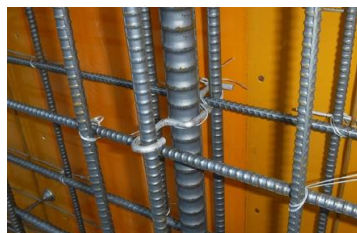
専用固定ジグ
