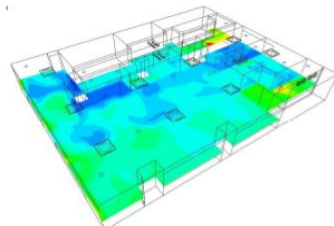
温度・湿度シミュレーション
