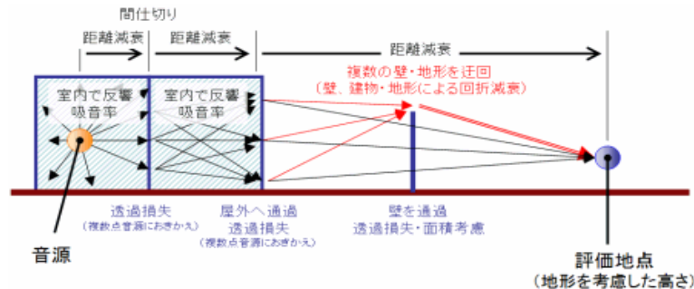
音環境のシミュレーション
