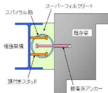
接合部断面
