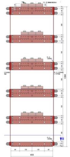
振動模型案(5層耐震モデル)
